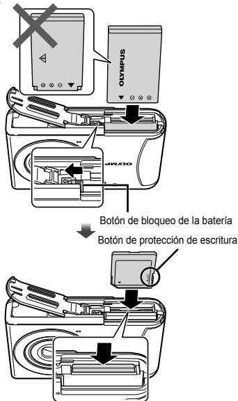
Tapa del compartimento de la batería/tarjeta
