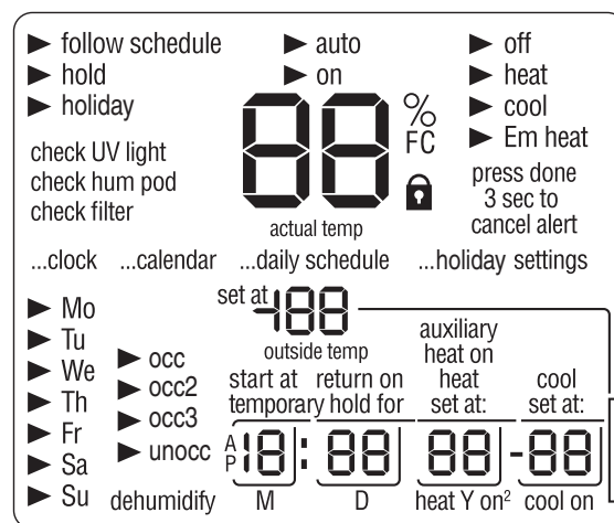
Fig. 1 — Thermostat Display
